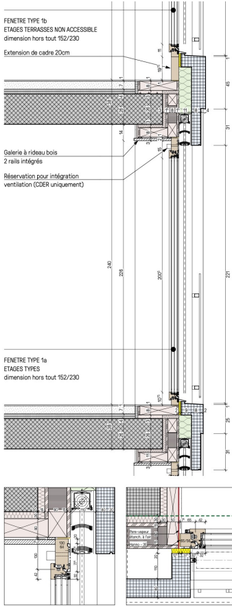
Détail type façade logements Cité Derrière / SILL
